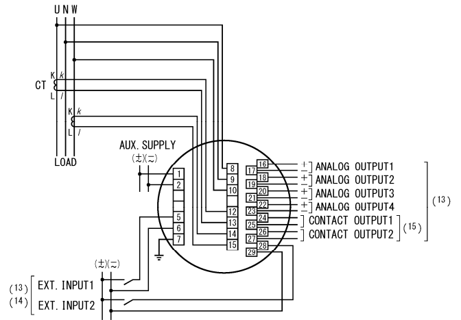
(2) 1φ3W
