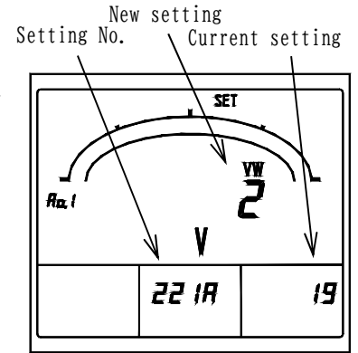
Ao1 output element
