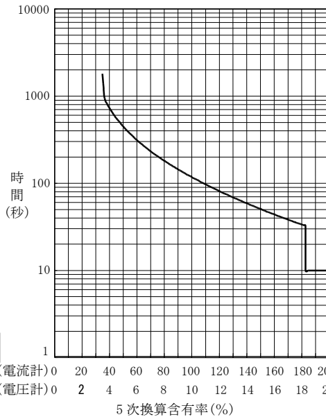
警告出力 反限時特性 上限設定値 35% (電圧計 3.5%) の場合
