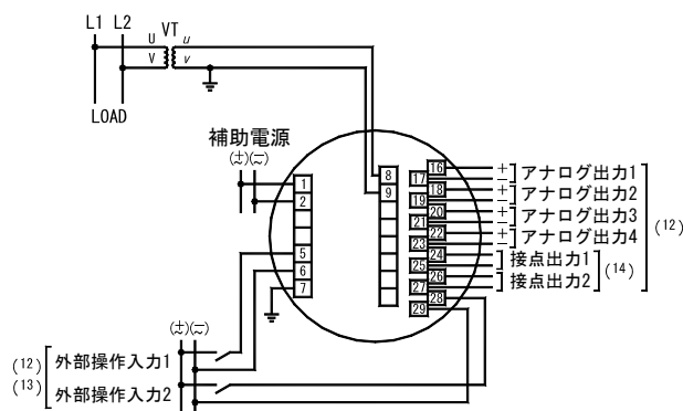
(11) 電圧入力 1φ2W
