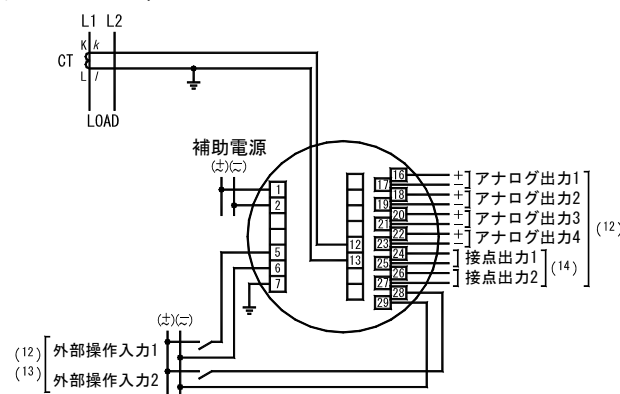
(8) 電流入力 1φ2W
