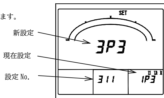
設定モード3 (No. 311 入力回路相線切替)
