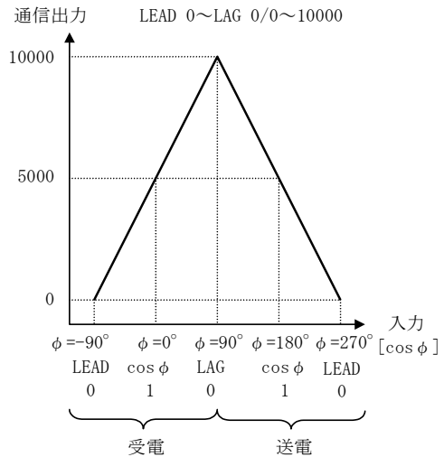
潮流計測
