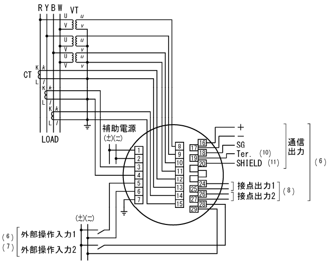
(2) 電圧，電流入力(3VT, 3CT)
