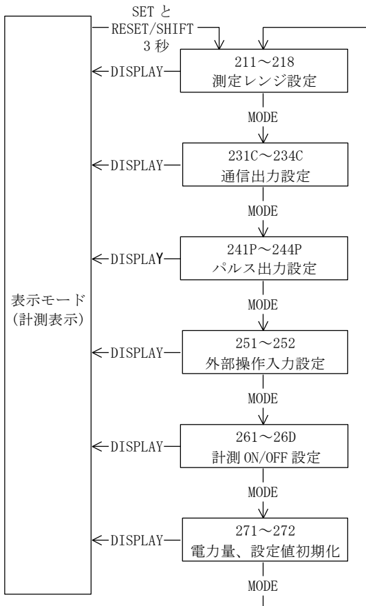
設定モード 2
