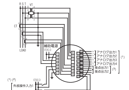
図-4 三相3線 (2VT, 3CT)
