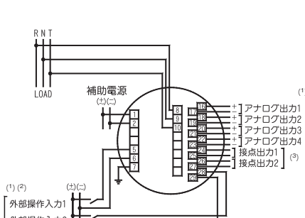
図-11 単相3線
