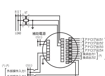
図-12 三相3線
