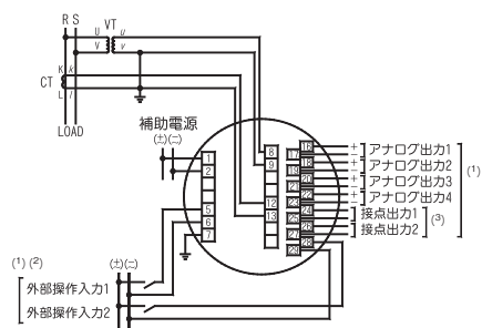
図-1 単相2線
