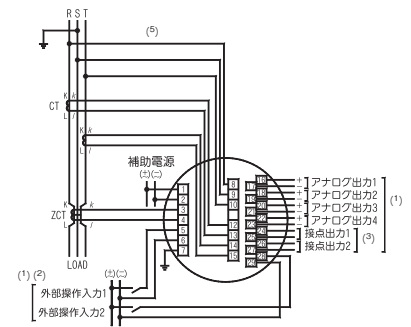
図-18 三相3線(S相接地)
