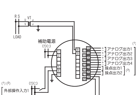
図-10 単相2線
