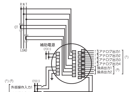
図-2 単相3線
