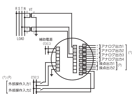
図-22 電圧入力 三相4線(2VT)
