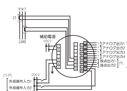
図-6 単相3線
