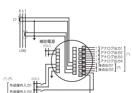
図-7 三相3線 (2CT)
