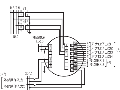
図-23 電圧入力 三相4線(3VT)
