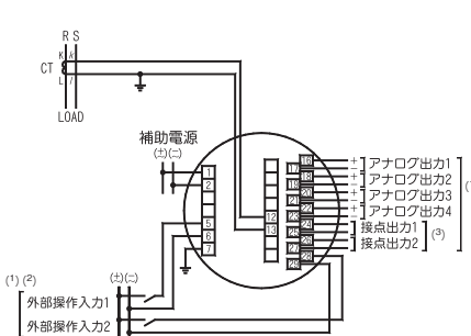
図-5 単相2線
