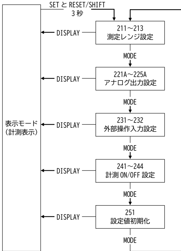
設定モード 2
