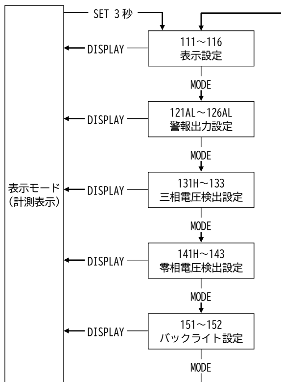
設定モード 1
