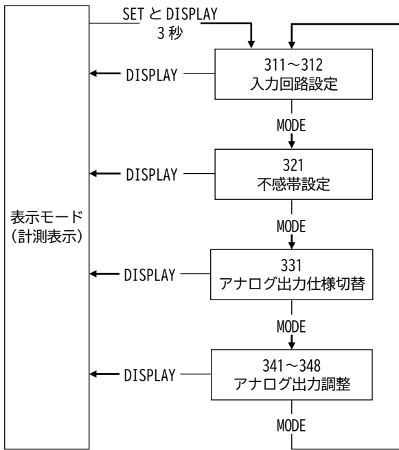
設定モード 3
