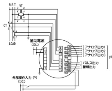
3φ3W(2VT, 2CT) アナログ出力 (6)
