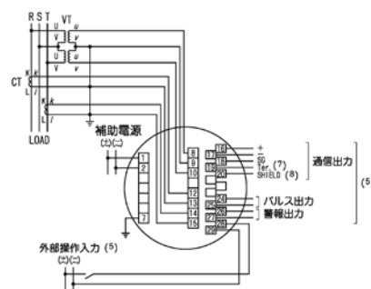
3φ3W(2VT, 2CT) 通信出力 (6)
