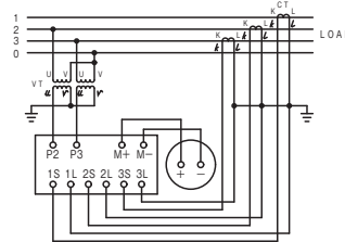
三相4線不平衡力率計 PPBD-96-34 PT-64M-34外付
