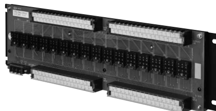
FWBS-16PN-00 480×130×40mm/1.6kg
